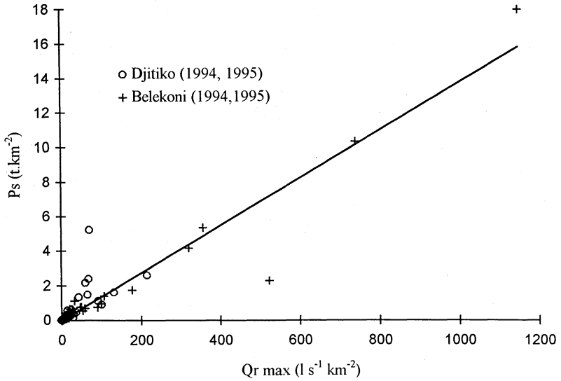
Fig. 3 Relation entre le poids de MES exporté ( P_s ) et le débit maximum ruisselé ( Q_r \text{ max} ) au cours des différentes crues observées à Djitiko et à Belekoni.
