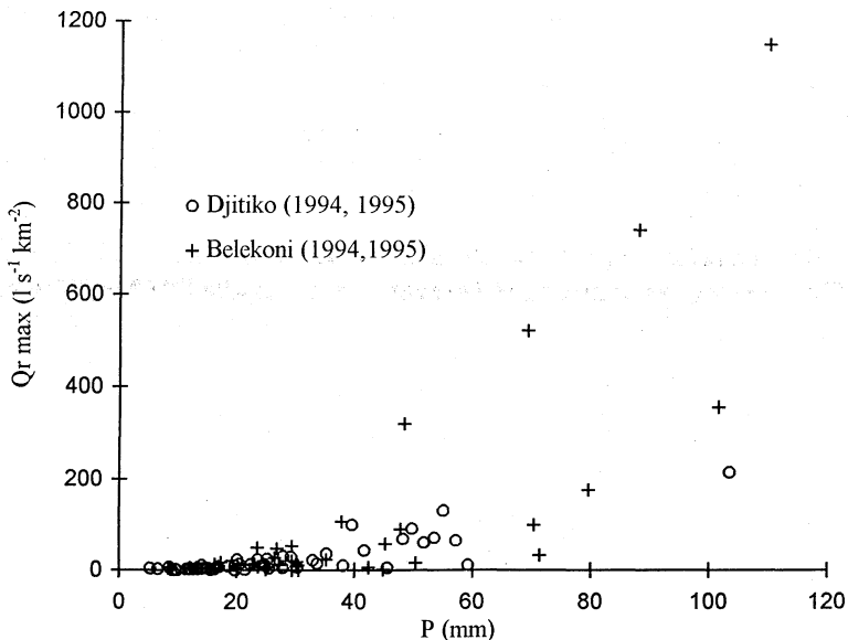
Fig. 2 Relation entre le débit maximum ruisselé ( Q_r \text{ max} ) et la pluie ( P ) au cours des différentes crues observées à Djitiko et à Belekoni.
