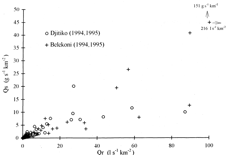
Fig. 4 Relation entre le débit solide moyen ( Q_s ) et le débit moyen de ruissellement ( Q_r ) au cours des différentes crues observées à Djitiko et à Belekoni.
