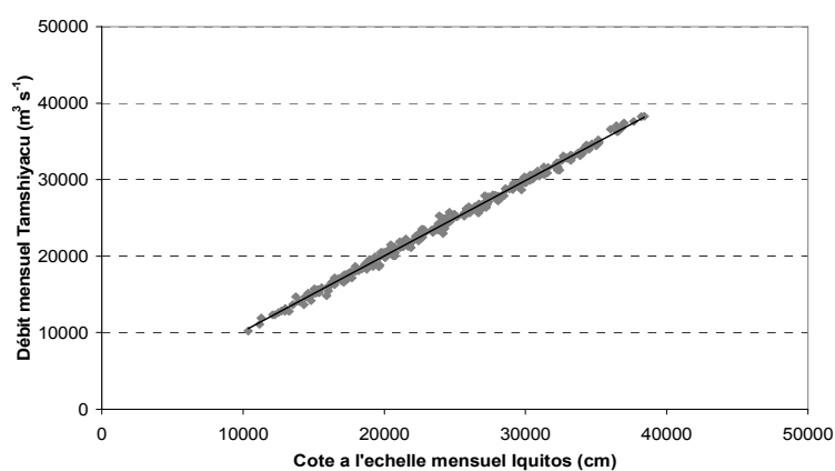
Fig. 3 Corrélation entre hauteurs d'eau mensuelles à Iquitos et débits mensuels à Tamshiyacu ( r^2 = 0.996 ) sur le Rio Amazonas.
